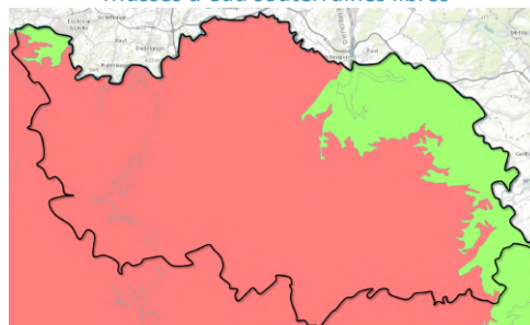
État chimique des masses d'eau souterraines (source : SDAGE 2022-2027)
