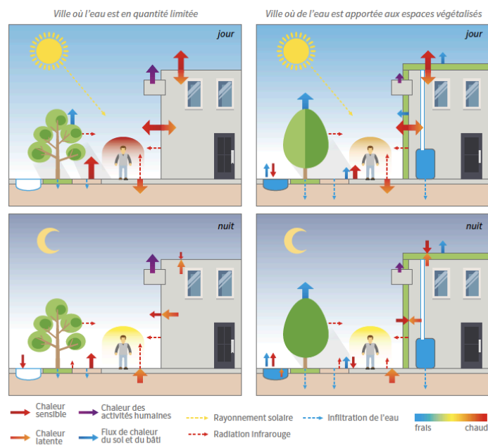
Les processus locaux du rafraîchissement urbain en été dans des villes. Source : Coutts et al., 2014 [9]
